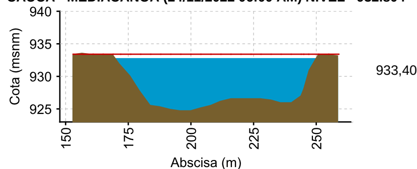
CAUCA - MEDIACANOA (24/11/2022 06:00 AM) NIVEL= 932.804
