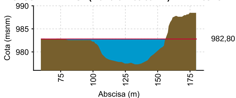
CAUCA - LA Balsa (24/11/2022 06:00 AM) NIVEL= 982.87
