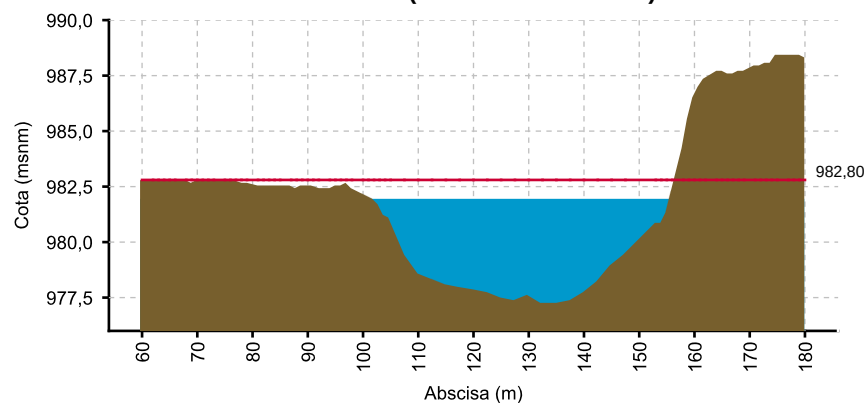
CAUCA - LA BALSA (08/06/2021 06:00 AM) NIVEL= 981.89
