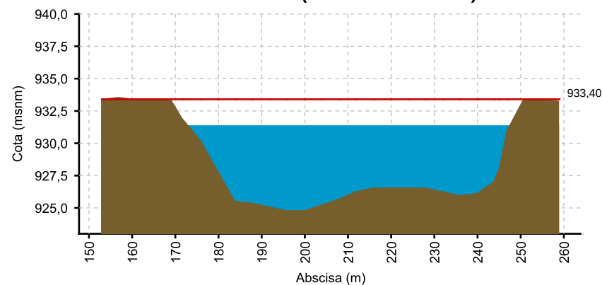
CAUCA - MEDIACANOA (03/06/2021 06:00 AM) NIVEL= 931.354
