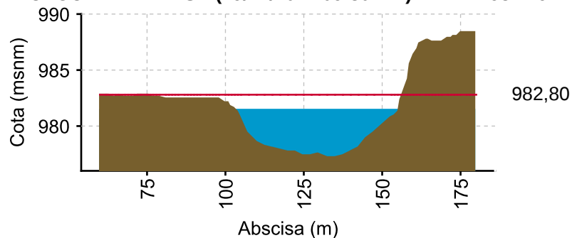
CAUCA - LA Balsa (19/12/2022 09:30 AM) NIVEL= 981.46
