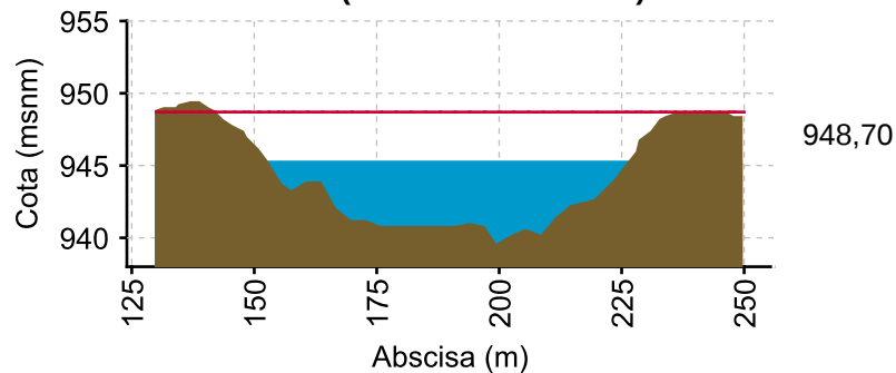
CAUCA - JUANCHITO (19/12/2022 04:00 PM) NIVEL= 945.333
