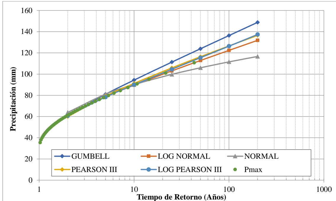
Figura 1.15. Precipitaciones máximas para los diferentes periodos de retorno. Estación El Aguacate
