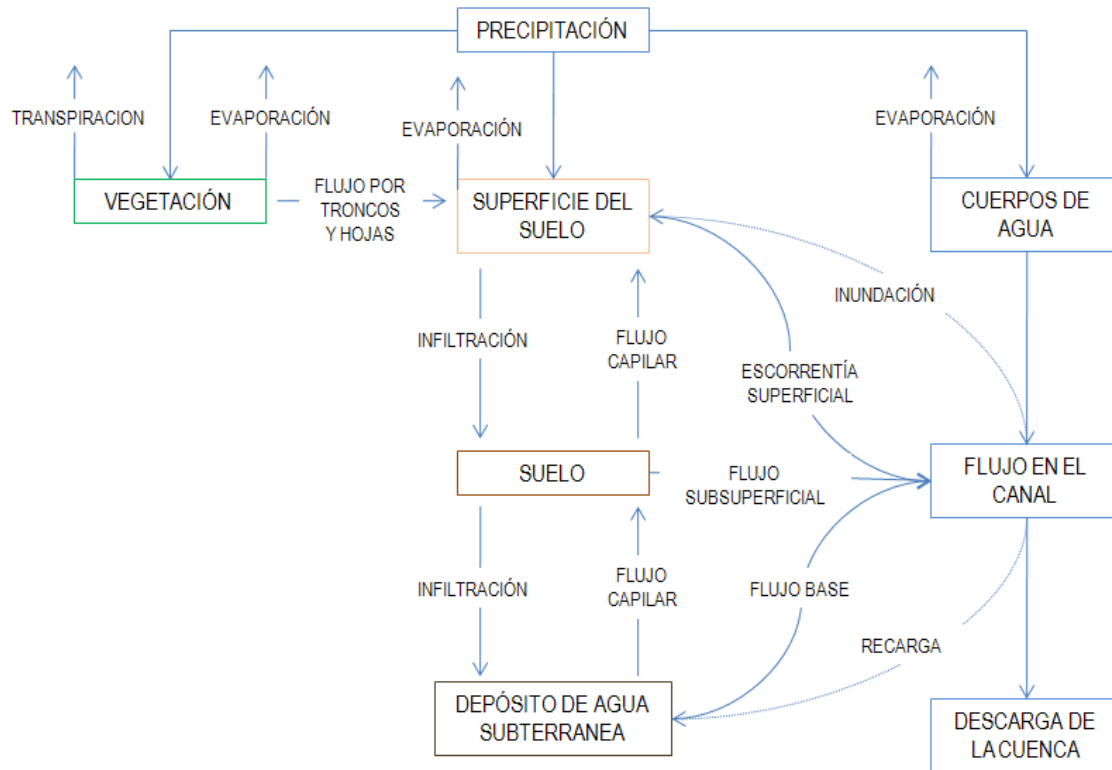
Figura 2.1. Esquema de las componentes hidrológicas e hidráulicas que utiliza el HEC-HMS 4.1.0 para representar una cuenca hidrográfica. Fuente. Adaptado de HEC, 2000
