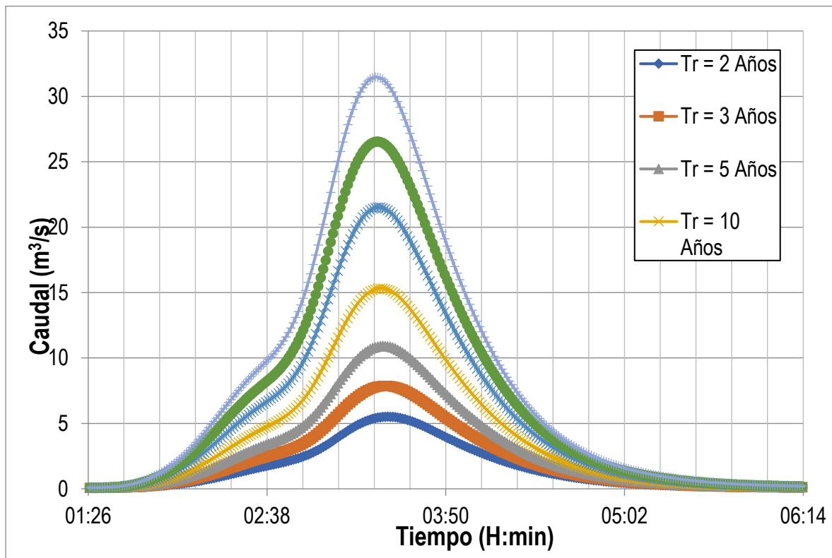
Figura 2.3. Hietograma e Hidrograma de caudales máximos para periodos de retorno de 2, 5, 10, 25, 50 y 100 Años zanjón Guabineros
