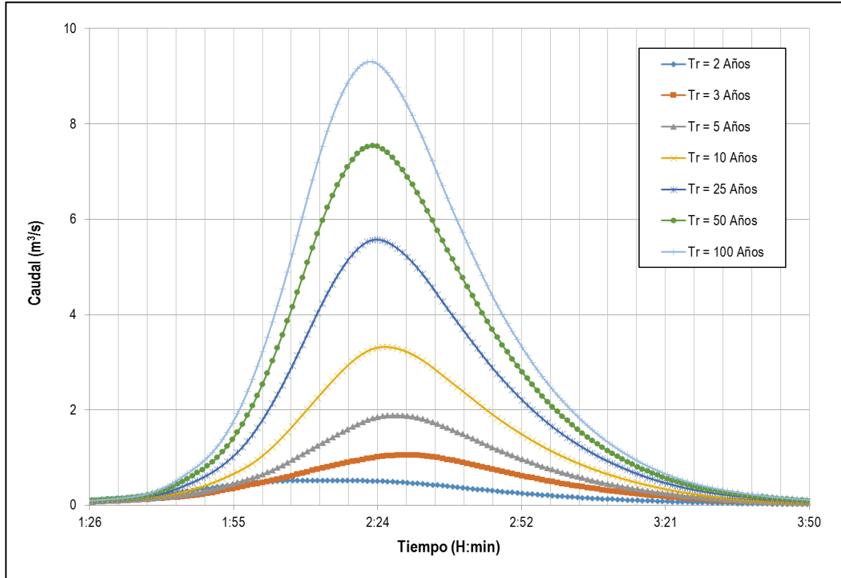
Figura 2.5. Hietograma e Hidrograma de caudales máximos para periodos de retorno de 2, 5, 10, 25, 50 y 100 Años zanjón El Rincón
