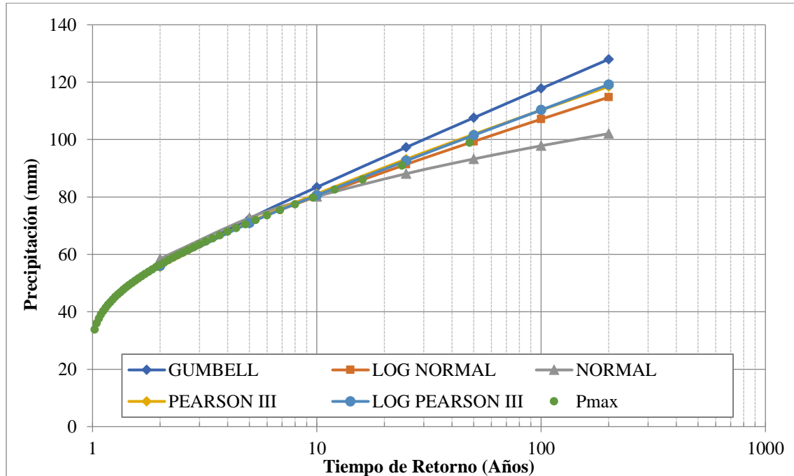
Figura 1.14. Precipitaciones máximas para los diferentes periodos de retorno. Estación La Herradura
