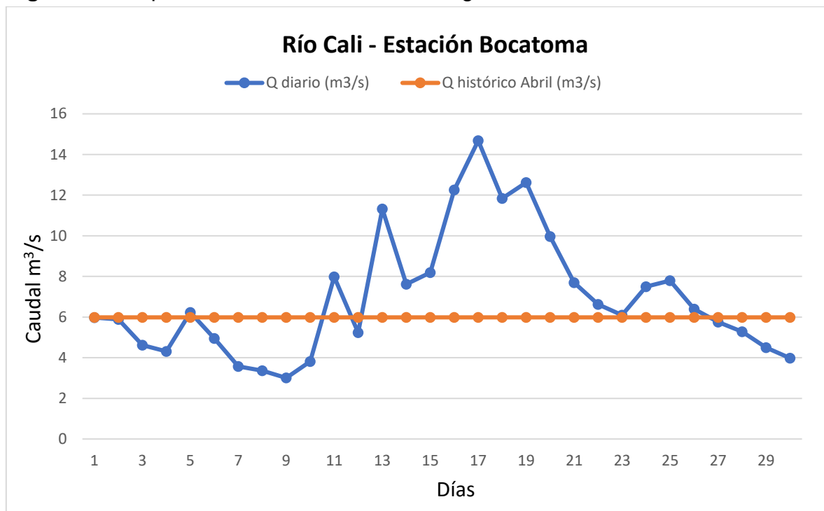
Figura 2. Comportamiento de la estación limnográfica Río Cali – estación Bocatoma.
