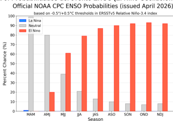
Figura 3: Probabilidades del evento ENOS (El Niño Oscilación del Sur).
